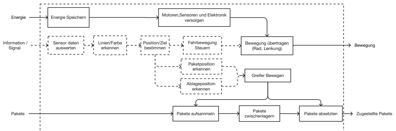
Abbildung 2: Funktionsstruktur
